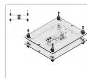
Válcový systém s osmibodovým uložením - nevyžaduje transportní pojistky a opakované kalibrace
