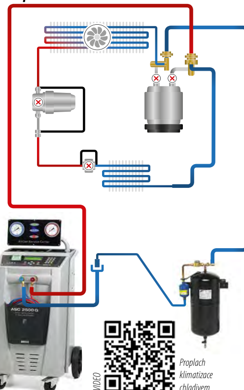
Tlaková nádoba na odpadní plyny Přípojovací hadice s nízkotlakou spojkou Kondenzace odpadních plynů přímo do nádoby neumožňuje monitorovat průběh kondenzace
